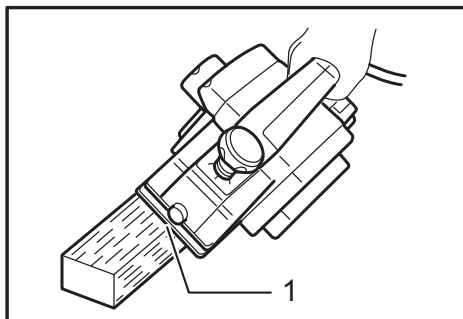
► 1. Alignez la rainure (Y) sur le bord de la pièce
