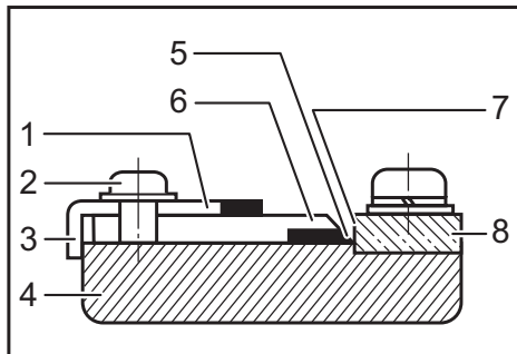
► 1. Placa de ajuste 2. Tornillos 3. Talón de la placa de ajuste 4. Lado trasero de la base del calibrador 5. Filo de cuchilla de corte 6. Cuchilla del cepillo 7. Borde interior de la placa calibradora 8. Placa calibradora
