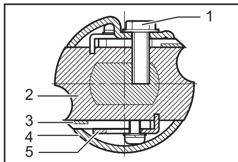
► 1. Perno 2. Tambor 3. Cuchilla del cepillo 4. Cubierta del tambor 5. Placa de ajuste
