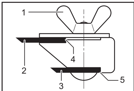
► 1. Écrou à oreilles 2. Rabot (A) 3. Rabot (B) 4. Côté (C) 5. Côté (D)
