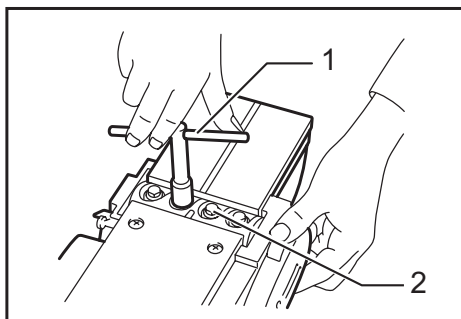
► 1. Clé à douille 2. Boulon de pose
