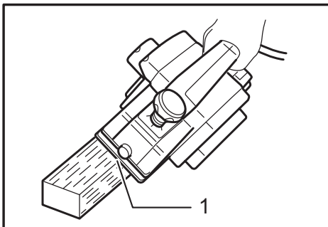
► 1. Alinear la ranura (Y) con la orilla de la pieza de trabajo
