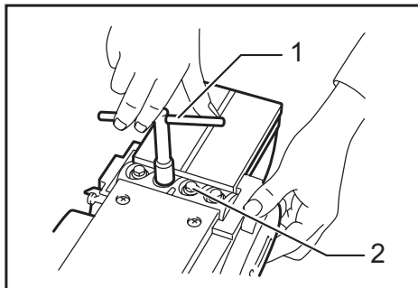
► 1. Llave de cubo 2. Tornillo de instalación
