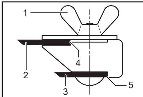
► 1. Tuerca de mariposa 2. Cuchilla (A) 3. Cuchilla (B) 4. Lateral (C) 5. Lateral (D)
