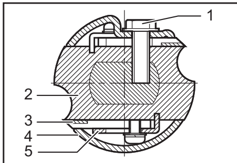
► 1. Boulon 2. Bloc de coupe 3. Fer de rabot 4. Contre-fer 5. Plaque de réglage
