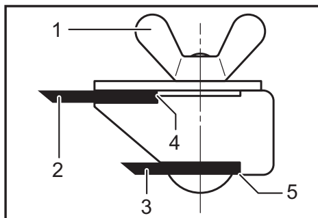
► 1. Wing nut 2. Blade (A) 3. Blade (B) 4. Side (C) 5. Side (D)
